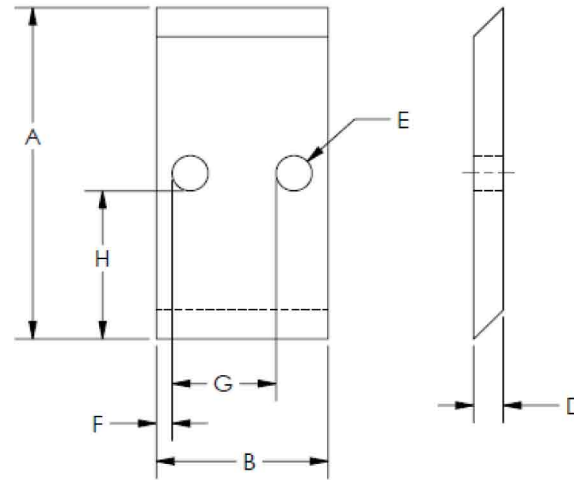
Double Bevel
